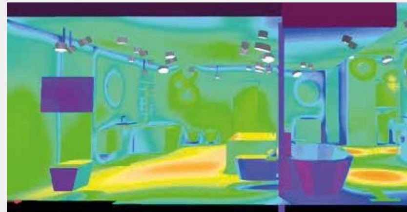
2. Расчет освещенности. Фиктивные цвета
